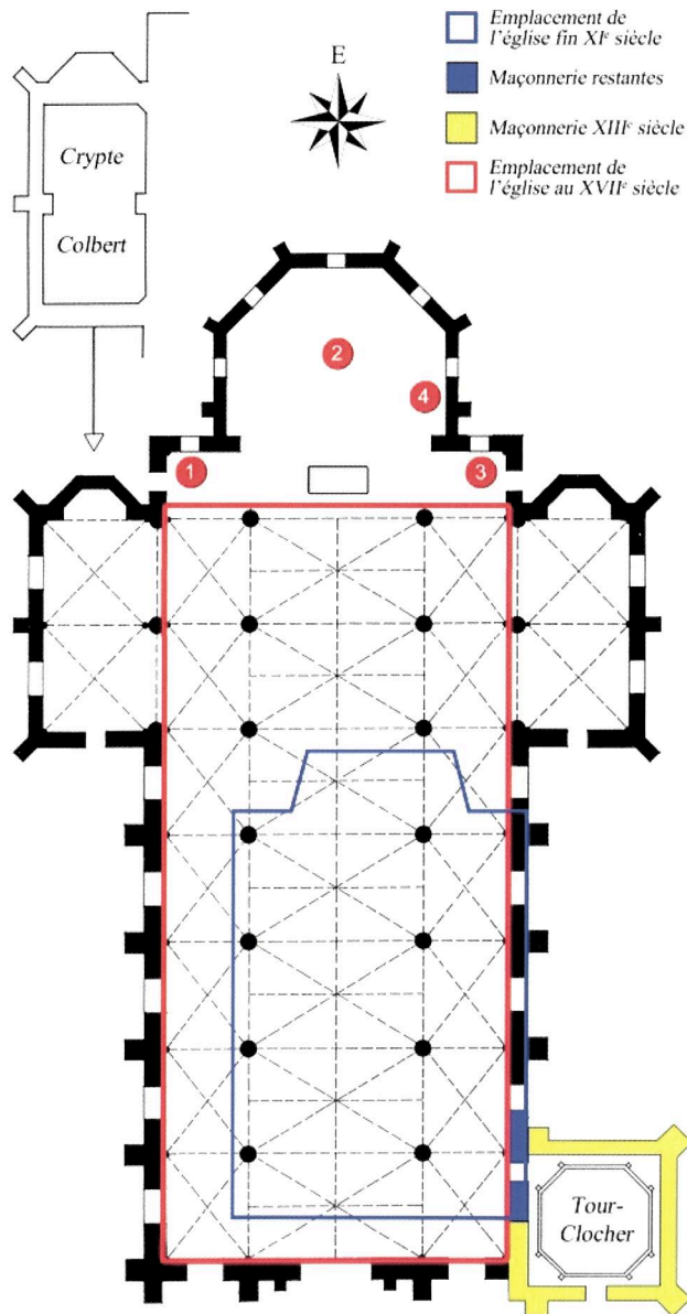
Vue en plan (Echelle : 1/400)
